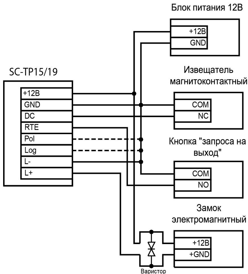
Рисунок 3. Схема подключения контроллера
